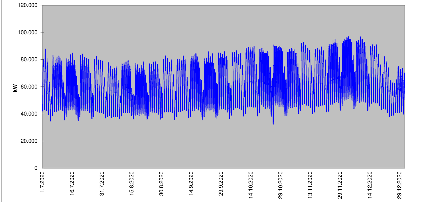
Summenlast der Einspeisungen Juli 2020 bis Dezember 2020
