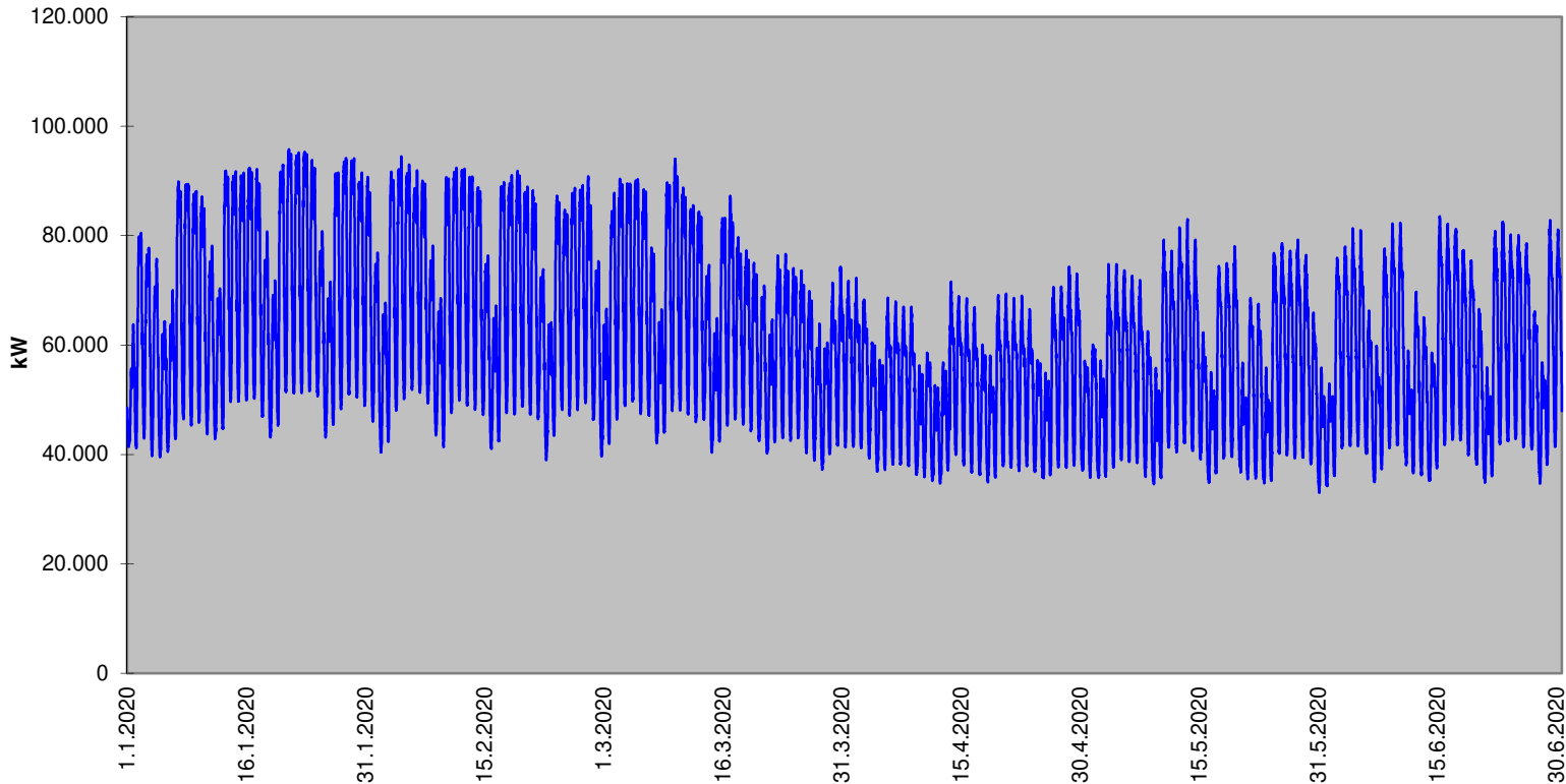
Summenlast der Einspeisungen Januar 2020 bis Juni 2020
