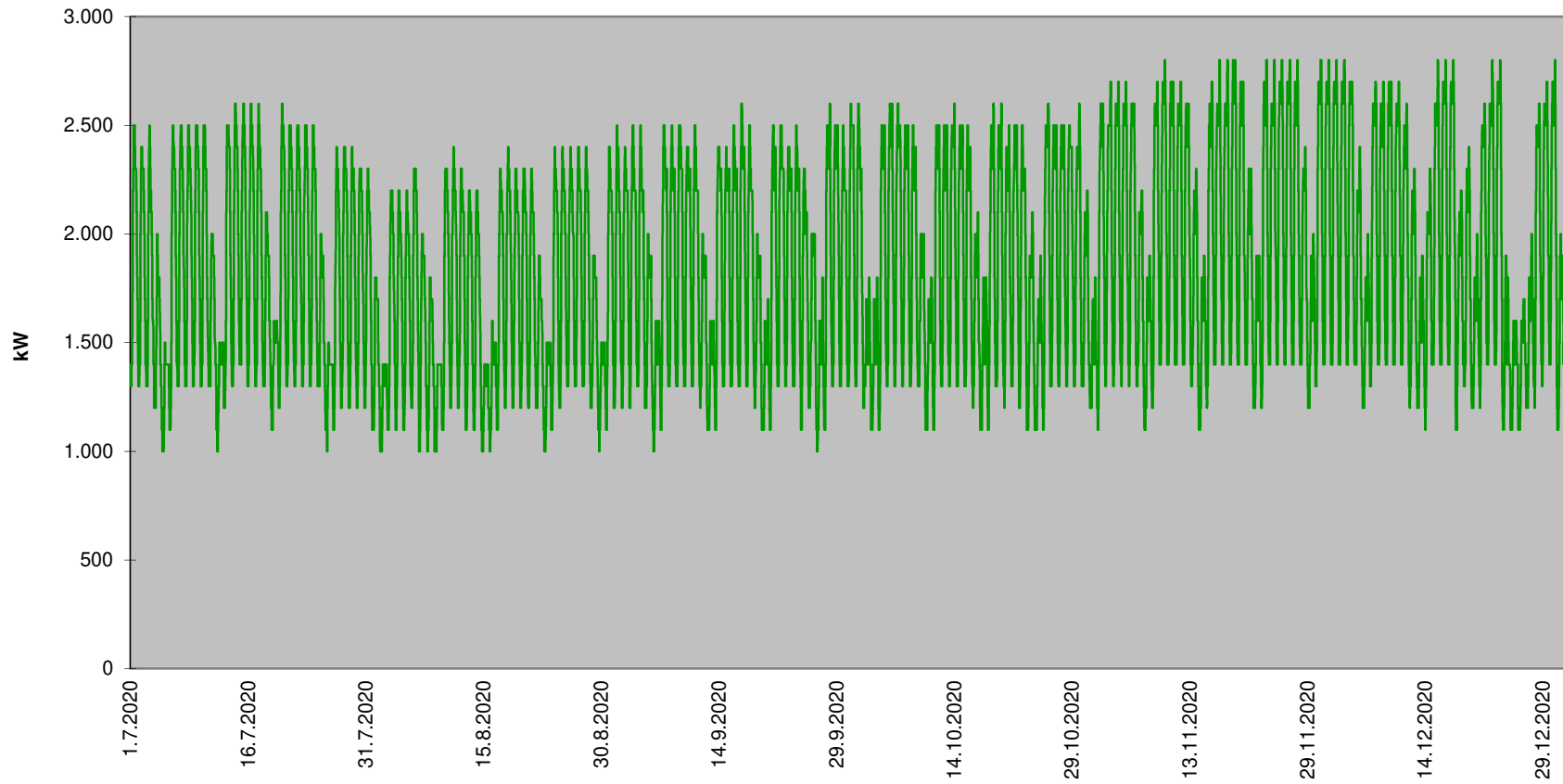
Lastganglinie der Gesamtverluste Juli 2020 bis Dezember 2020
