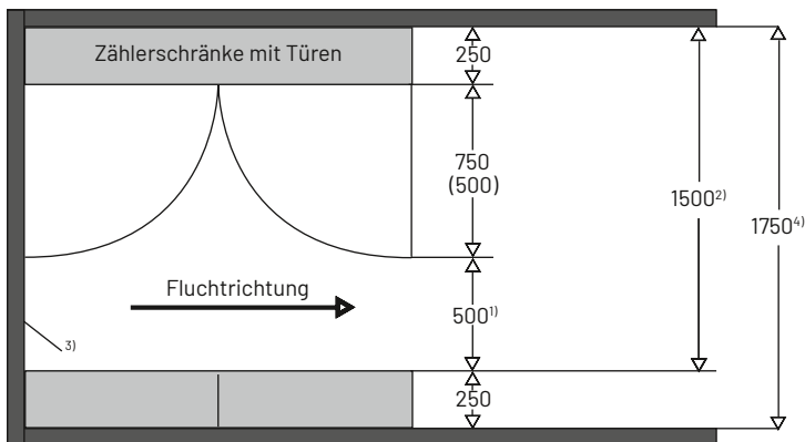
Abb. 2: Abmessungen eines Hausanschlussraums
